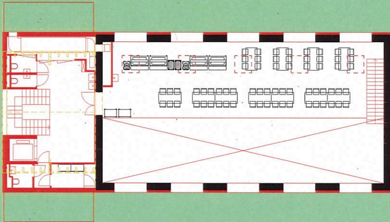
Grundriss 1. Obergeschoss
