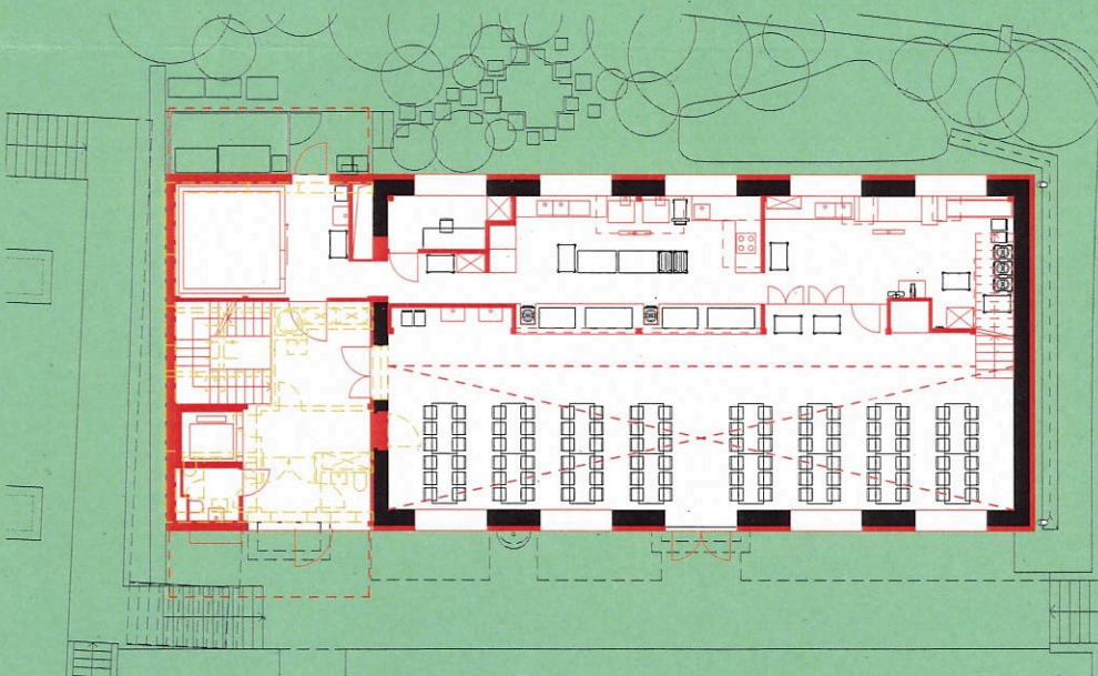
Grundriss Erdgeschoss
