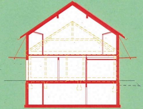
Querschnitt
