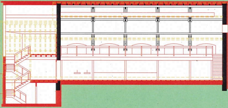
Längsschnitt
